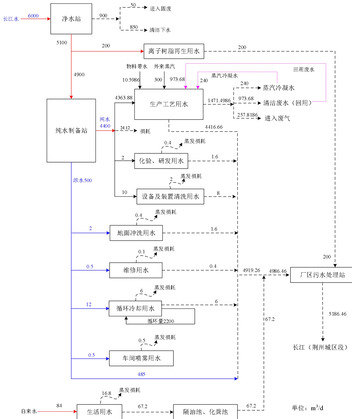
图 3-12 项目第二阶段、第三阶段均新增水平衡分析图 单位：m 3 /d
