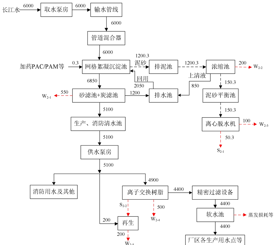
图 3-8 各阶段给电站及软电站物料平衡图 单位：m 3 /d
