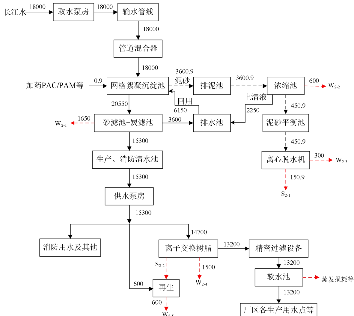
图 3-9 项目全部建成后全厂给电站及软水站物料平衡图 单位：m 3 /d
