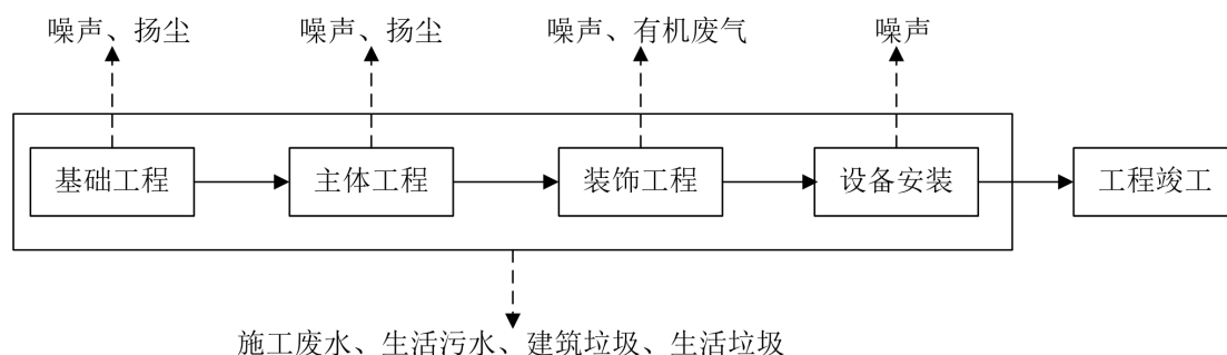
图 3-18 项目施工期工艺流程及产污环节图
