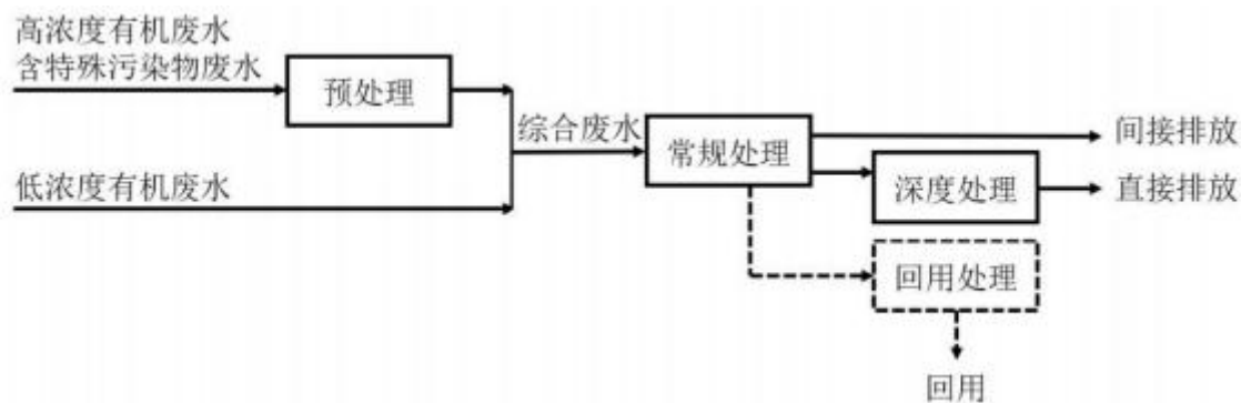
图 7-2 纺织染整工业废水处理工艺流程示意图
