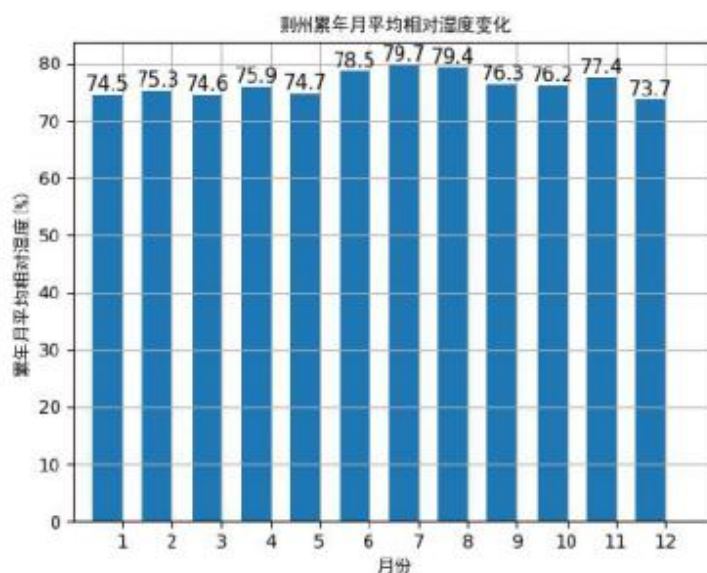
图 5-10 荆州月平均相对湿度（纵轴为百分比）
