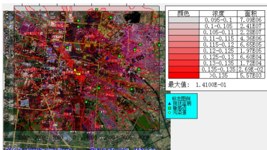
TVOC 1 小时浓度叠加值
