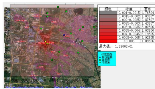
NH 3 1 小时浓度贡献值
