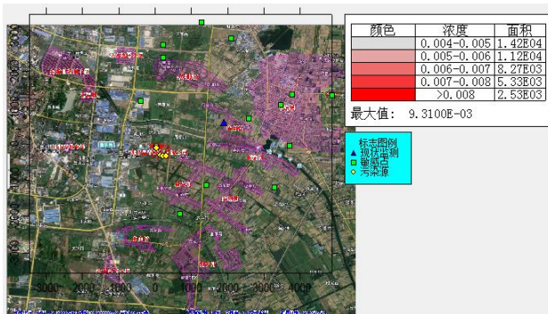
H 2 S 1 小时浓度叠加值
