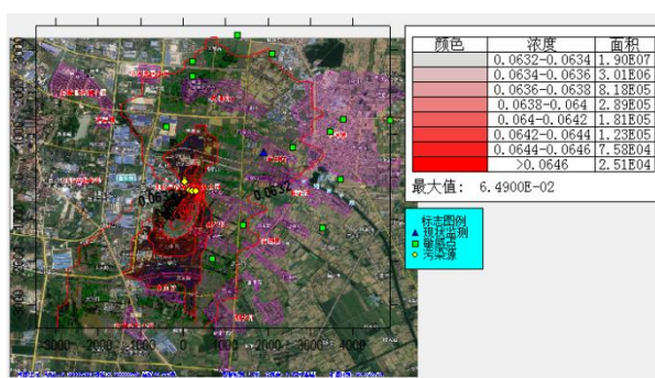
PM 10 年平均浓度叠加值
