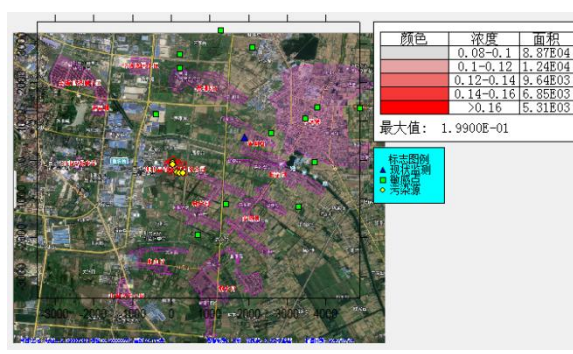
NH 3 1 小时浓度叠加值
