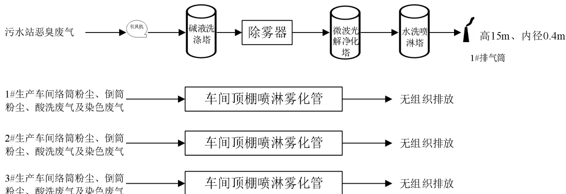
图 7-1 项目废气治理措施示意图
