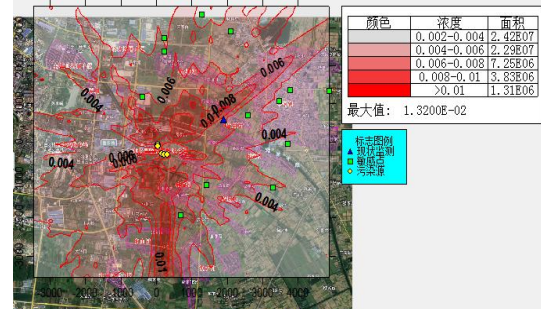
TVOC 8 小时浓度贡献值
