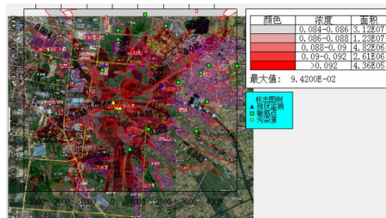
TVOC 8 小时浓度叠加值
