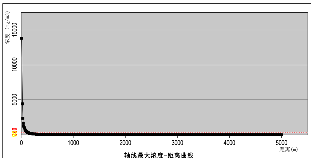
图 6-11 最常见气象条件下，下风向不同距离处，CO 最大浓度分布图
