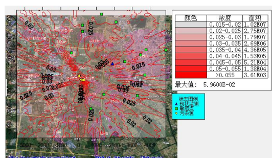
TVOC 1 小时浓度贡献值
