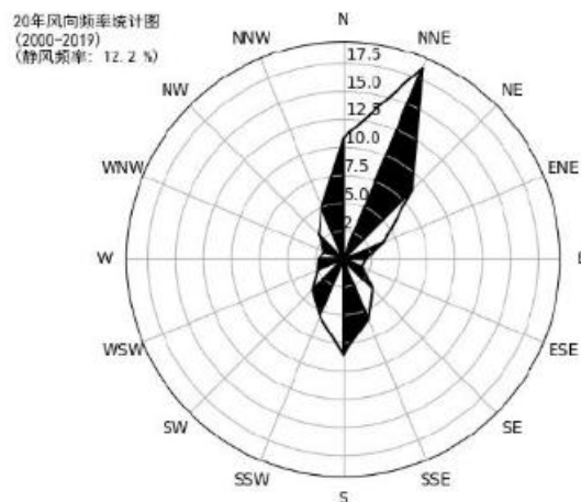
图 5-1 荆州风向玫瑰图 (静风频率 12.2%)
