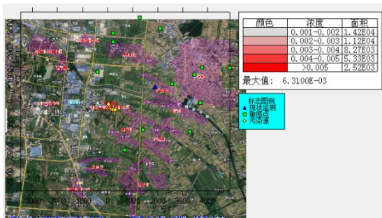
H 2 S 1 小时浓度贡献值
