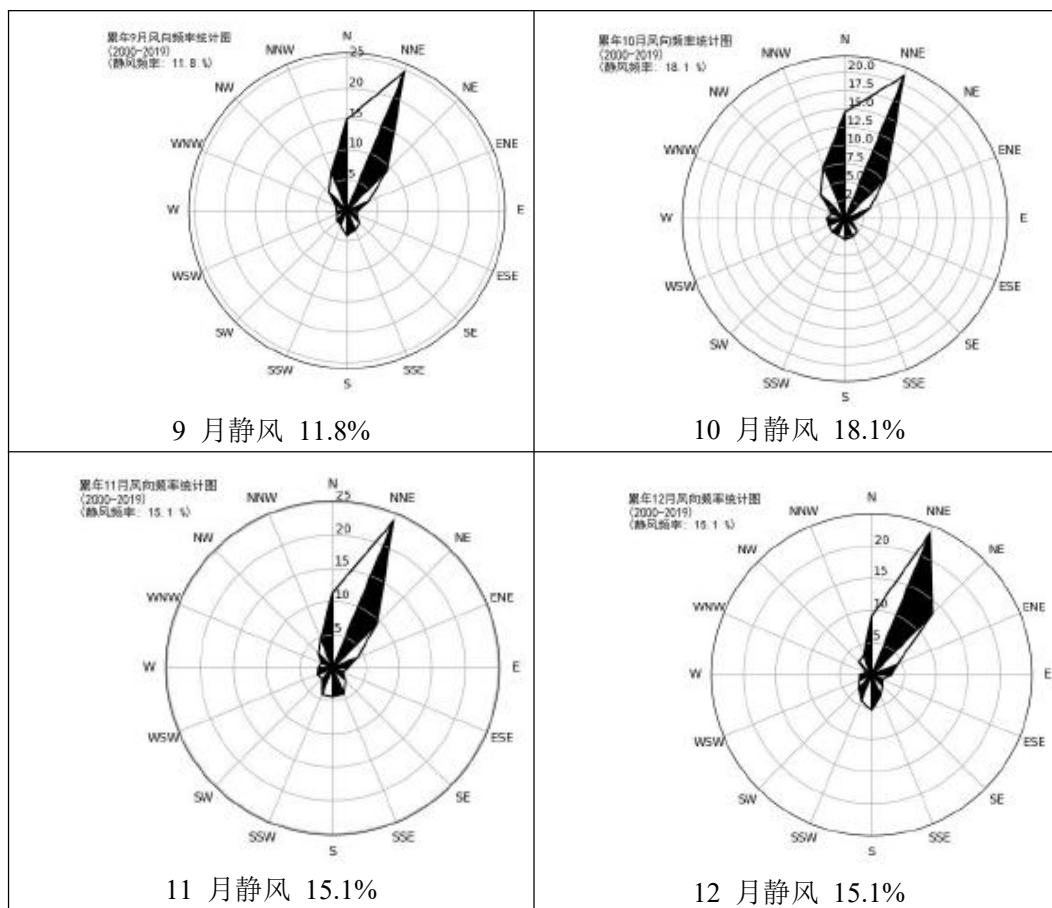
图 5-2 荆州月风向玫瑰图
