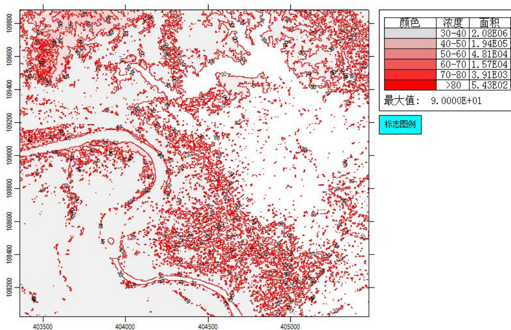
图 5-12 预测范围等高线示意图
