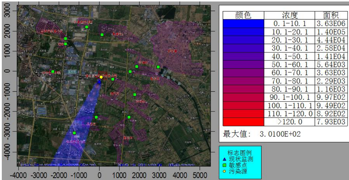
图 6-3 最不利气象条件下，醋酸各网格点浓度分布图
